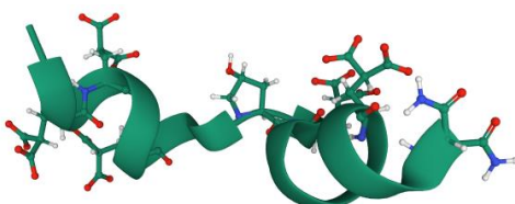
شکل ۳۱) ساختار روبانی کونانتوکین-RiB Fig 31) Conantokin-RiB ribbon structure
