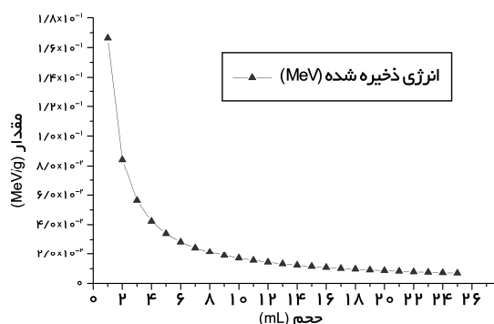
(b) دوز جذبی بتا در تیروئید برای ۱۳۱ید (ارگان چشمه، غده تیروئید بوده است).
