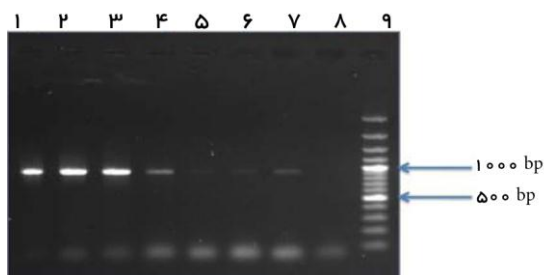
شکل ۲) آزمایش تعیین حساسیت برای رقت‌های مختلف DNA تخلیص شده سرووار L. Canicola (۱): ۱۰ ng؛ (۲): ۱ pg؛ (۳): ۱۰۰ pg؛ (۴): ۱۰ pg؛ (۵): ۵ pg؛ (۶): ۲ pg؛ (۷): ۱ pg؛ (۸): ۱ pg؛ (۹): ۰/۱ سائیز مارکر
