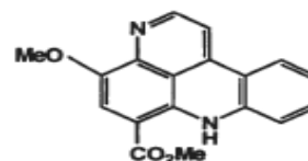
norsegolone
