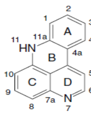
پیریدواکریدین
