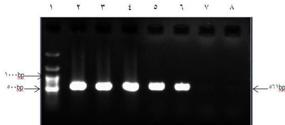
شکل (۱) نتایج الکتروفورز محصولات PCR نمونه‌های بیماری‌زا و غیربیماری‌زا بر روی ژل آگارز ۱ درصد (۱) سایز مارکر، سرووارهای (۲) کانیکولا، (۳) پومونا، (۴) سرجهاردجو، (۵) ایکتره‌موراژی، (۶) گریپتوفوزا (نمونه‌های مثبت)، (۷) سرووار غیربیماری‌زای بایفلکسا (منفی)، (۸) کنترل منفی
