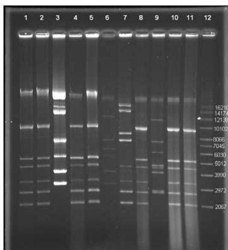
شکل ۱) الگوی پلاسمیدی ۱۱ سویه از پسودوموناس آئروژینوزای. چاهک شماره ۱ دو سویه با الگوی یکسان، چاهک ۳ سویه با الگوی متفاوت، چاهک ۴ و ۵ دو سویه با الگوی یکسان، چاهک ۶، ۷، ۸، ۹ و ۱۰ چهار الگوی متفاوت، چاهک ۱۰ و ۱۱ دو الگوی یکسان، چاهک ۱۲ مارکر (Supercoiled DNA Ladder).
