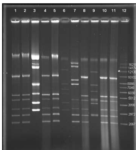
شکل ۱) الگوی پلاسمیدی ۱۱ سویه از پسودوموناس آئروژینوزای. چاهک شماره ۲ دو سویه با الگوی یکسان، چاهک ۳ سویه با الگوی متفاوت، چاهک ۴ و ۵ دو سویه با الگوی یکسان، چاهک ۶، ۷، ۸ و ۹ چهار الگوی متفاوت، چاهک ۱۰ و ۱۱ دو الگوی یکسان، چاهک ۱۲ مارکر (Supercoiled DNA Ladder).
