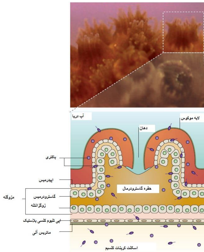
شکل ۱) ساختار بافت مرجان. مرجان‌های سخت متشکل از سه ساختار هستند که برای باکتری‌ها زیستگاه مناسب مهیا می‌کند: لایه موکوس سطحی، بافت مرجان (حفره گاسترودرمال) و اسکلت کربنات کلسیم. زوگزائتله در گاسترودرمیس جای دارند (۱۶).
