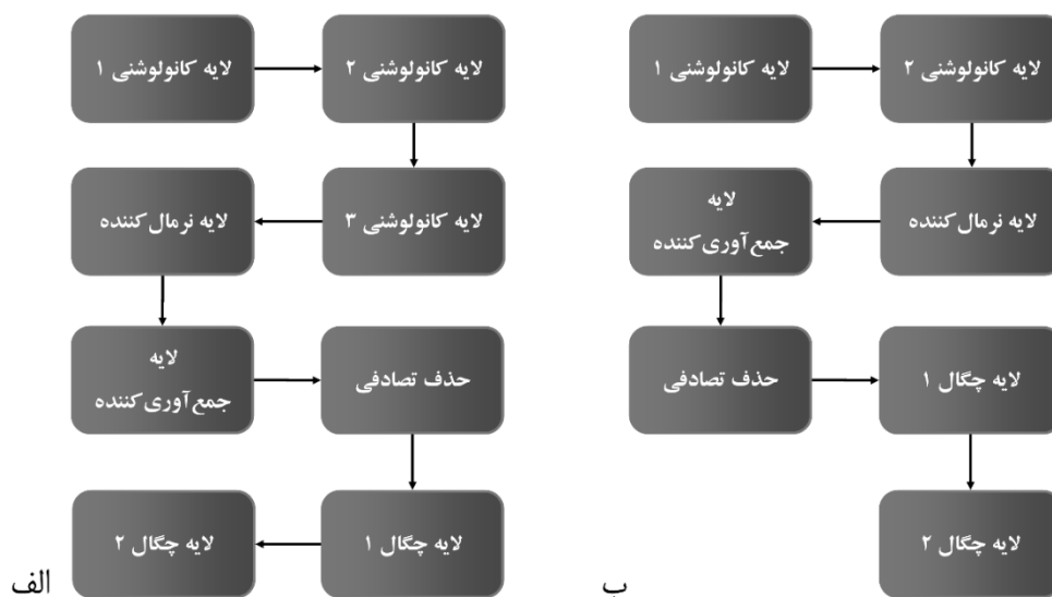
شکل ۴) ساختارهای مختلف بررسی شده برای شبکه عصبی کانولوشنی: در این پژوهش ساختارهای متفاوتی از شبکه‌های عصبی کانولوشنی با تعداد لایه‌های متفاوت برای مقایسه کارایی آنها در فرایند طبقه‌بندی گلوبول‌ها مورد بررسی قرار گرفته‌اند که دو نمونه از این ساختارها در این شکل نشان داده شده است؛ الف: ساختار با سه لایه کانولوشنی. ب: ساختار با دو لایه کانولوشنی.
