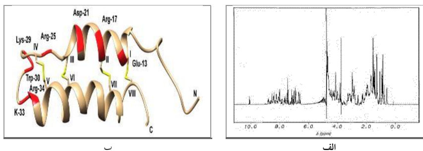
شکل ۱۲ الف: طیف ^1\text{H-NMR} یک‌بعدی در ۵۰۰ مگاهرتز توکسین B-IV (۱۳۹). ب: ساختار ^1\text{NMR} توکسین (B-IV) شناسه RCSB: VIB (۱۴۰)؛ رنگ قرمز: بقایای مهم برای فعالیت؛ عدد رومی: بقایای Cys؛ رنگ زرد: پیوندهای دی‌سولفیدی
