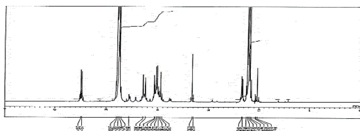
شکل ۹) طیف ^1\text{H-NMR} توکسین جدا شده از کرم سفالوتریکس سیمولای خلیج هیروشیما. استفاده از پنج میلی گرم HMT در نیم میلی‌لیتر \text{CD}_3\text{COOD} یک درصد در \text{D}_2\text{O} . برای تعیین طیف ^1\text{H-NMR} توسط طیف سنج JNM-500 NMR و استون به‌عنوان استاندارد داخلی (۱۲۵).
