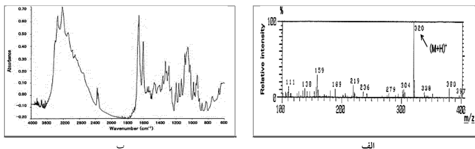
شکل ۸) الف: طیف جرمی یونیزاسیون الکترواسپری از توکسین (HMT) جدا شده از کرم روبان گونه سفالوتریکس در خلیج هیروشیما توسط طیف سنج جرمی ESI-MS؛ ب: طیف IR از این توکسین توسط FT-IR، مجهز به میکروسکوپ FT-IR (۱۲۵).
