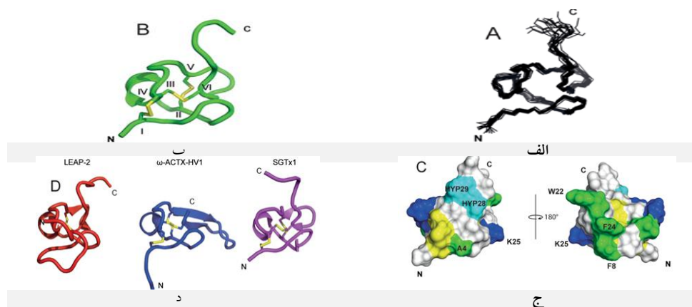
شکل ۱۸). ساختار NMR نمرتیدهای \alpha -1 و شناسایی همولوگ‌های آن. (الف): نمایش خطی مدل با کمترین امتیاز MolProbity (ب): نمایش روبانی با دی سولفیدها (اعداد رومی)، C و N-ترمینال‌ها نمایش داده شدند. (ج): مدل سطحی. بقایای اساسی به رنگ‌های آبی؛ غیر قطبی به رنگ سبز؛ سیستین‌ها به رنگ زرد و هیدروکسی‌پرولین‌ها در سیان نشان داده شده‌اند. اسیدهای آمینه آروماتیک F8، F22 و W24، نشان‌دار هستند. اسیدهای آمینه F8 تنها تفاوت بین \alpha -1 و \alpha -2 است. ساختارها با استفاده از MOLMOL و PyMOL نمایش داده شده‌اند. شناسه PDB نمرتیدهای \alpha -1: 6ENA بود. (د): نزدیک‌ترین همولوگ ساختاری \alpha -1 مشخص شده از PDB با استفاده از Daliserver: پپتید ضد میکروبی بیان شده کبدی ۲ (LEAP-2, PBD: 2l1q-A)، \omega -آتراکوتوکسین HV1a- ۲۱۰ (SGTx1, PBD: 1la4-A) Scg1a- ۲۱۱ و K-ترافوتوکسین \omega -ACTX-HV1, PBD: 1axh-A).
