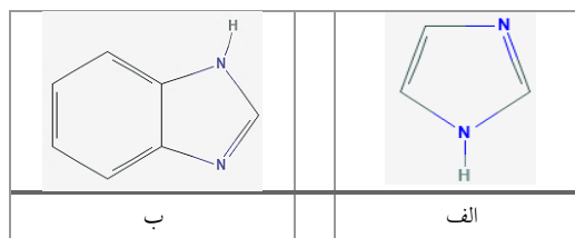
شکل ۵) ساختارهای هسته‌های ایمیدازولی (الف) و بنزایمیدازولی (ب) (منبع: پاکم ۲۸ ) Fig 5) Nucleous structures of imidazole (A), and benzimidazole (B) (Source: Pubchm)
