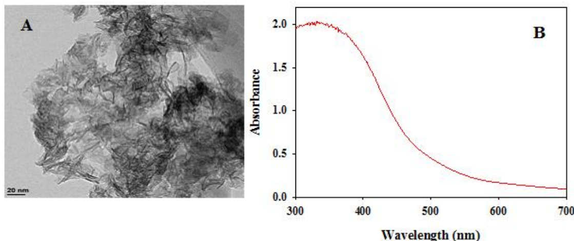
شکل ۲ (A) تصویر میکروسکوپ الکترونی نانوصفحات دی اکسید منگنز و (B) طیف ناحیه UV-vis نانوصفحات دی اکسید منگنز سنتز شده با صمغ عربی Fig 2) (A) TEM image of \text{MnO}_2 nanosheets and (B) UV-vis spectrum of \text{MnO}_2 nanosheets synthesized with Gum Arabic
