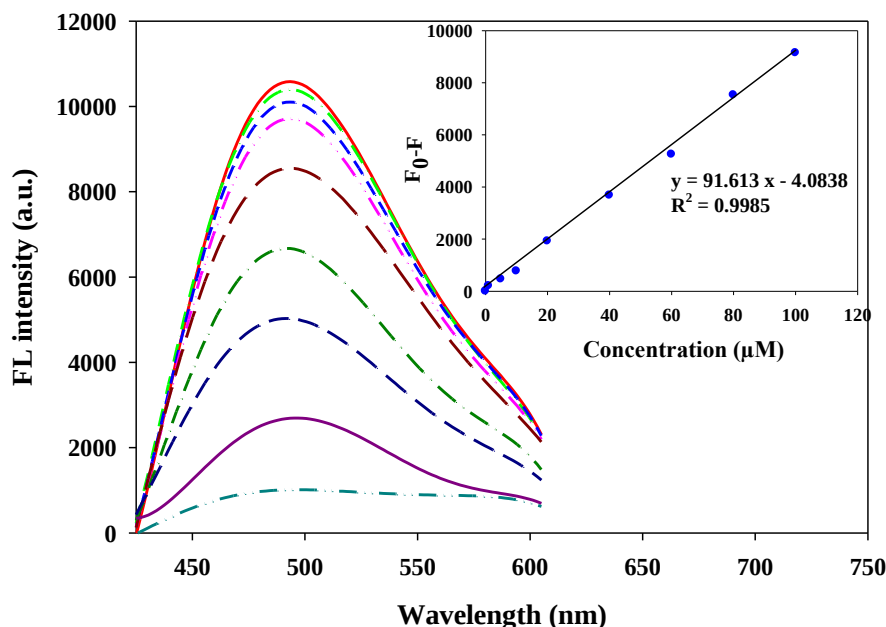
شکل ۷) طیف‌های نشر فلورسانس نانوذرات پلی دوپامین در حضور غلظت‌های مختلف گالیک اسید در محدوده ۰ تا ۱۰۰ میکرومولار. قسمت داخلی: رابطه بین مقادیر کاهش شدت سیگنال فلورسانس ( F_0-F ) در برابر غلظت گالیک اسید (منحنی کالیبراسیون)
