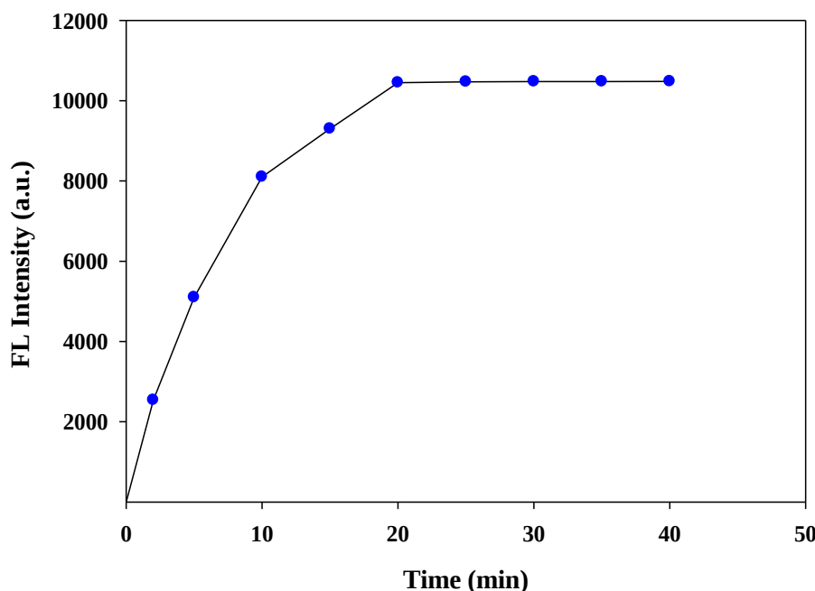
شکل ۵) زمان مورد نیاز برای واکنش بین دوپامین و نانوصفحات \text{MnO}_2 و تشکیل نانوذرات پلی دوپامین فلورسانس کننده
