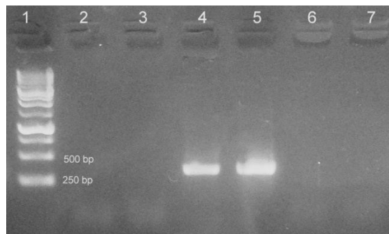
شکل ۶) نتیجه انجام واکنش کلونی PCR. باندهای اختصاصی با اندازه ۳۵۰ جفت باز در ستون‌های ۴ و ۵ قابل مشاهده است. ستون ۱ مارکر DNA و ستون ۶ کنترل منفی را نشان می‌دهد.
