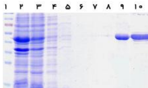
شکل ۲) بررسی مراحل تخلیص پروتئین نوترکین DnaK با استفاده از ژل ۱۲ درصد SDS-PAGE در آکریلامید در
