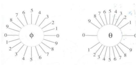
شکل (۱) روش Orientator برای به دست آوردن برش‌های تصادفی و همگون (IUR)
