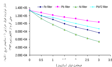
شکل ۴. شار نوترون فوق حرارتی بر حسب ضخامت فیلتر نوترونی
