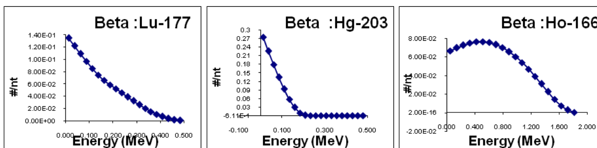
شکل (۲) طیف بتای ایزوتوپ‌های ^{203}\text{Hg} ، ^{177}\text{Lu} و ^{166}\text{Ho}
