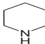
شکل ۴۲) ساختار پیپریدین
