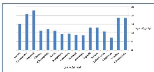
نمودار ۳) مقدار اسید چرب (C16:0) موجود در دریایی هولوتوریا اسکبرا ( H. Scabra ) در مطالعه اخیر، در مقایسه با دیگر مطالعات مورد بررسی
