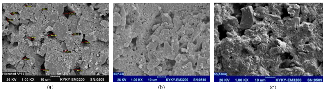
شکل ۵) تصویر میکروسکوپ الکترونی روبشی از سطح بسترهای فیلتر سرامیکی (a: سرامیک معمولی؛ b: بسترهای فیلتر سرامیکی پوشش‌دهی شده با نانوذرات نقره در حضور APTES، پس از ۱۸ ساعت غوطه‌وری در کلوئید نانوذرات نقره؛ c: بسترهای فیلتر سرامیکی پوشش‌دهی شده با نانوذرات نقره در حضور APTES، پس از ۲۴ ساعت غوطه‌وری در کلوئید نانوذرات نقره).
