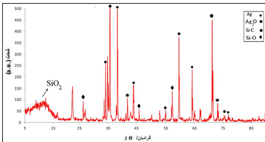
شکل ۳) طیف XRD بسترهای فیلتر سرامیکی پوشش‌دهی شده با نانوذرات نقره در حضور پیش ماده APTES، پس از ۲۴ ساعت غوطه‌وری در کلونید نانوذرات نقره
