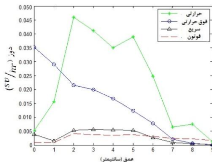
شکل ۱۰) دوز مؤثر نوترون و اشعه گاما در عمق‌های مختلف سر انسان. غلظت بور در تومور و بافت سالم مغز به ترتیب 40 \text{ ppm} و 10 \text{ ppm} می‌باشند.
