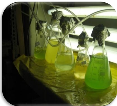
شکل ۳) پرورش ریز جلبک‌ها در شرایط مناسب
