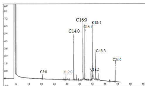
شکل ۶) کروماتوگرام حاصل از ترکیب اسیدهای چرب جلبک Chlorella sp.
