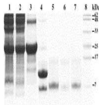
شکل ۳۲) آنالیز SDS-PAGE / تریس / تریسین rSN316، rSN311 و rSN285 لاین ۱: پروتئین تام pETTRXSN285-
