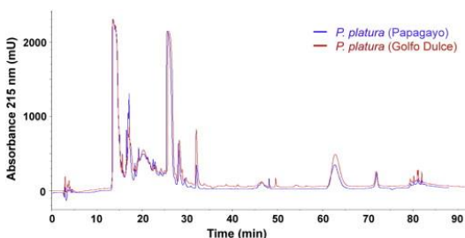
شکل ۱۵) مقایسه کروماتوگرام‌های مربوط به ونوم‌های پروتئینی نمونه‌های جمع‌آوری شده مار دریایی شکم‌زرد ( Pelamis platyura )، در دو منطقه کاستاریکا (خلیج پاپاگایو و خلیج دولک)، با HPLC فاز معکوس در یک ستون C 18
