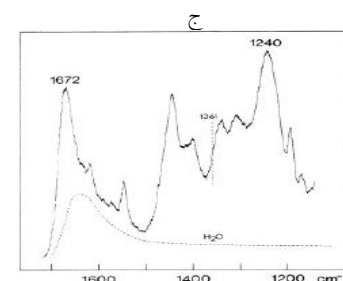
طیف رامان نوروتوکسین خالص جدا شده از زهر Lapemis hardwickii در محلول آبی در pH 7
