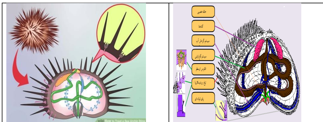
شکل (۳) شمای یک توتیای دریایی و برخی ارگان‌های مهم آن. تیغ (خار) و پدیسلا رین یکی ارگان‌های زهری و محل ونوم و برخی ترکیبات فعال زیستی.
