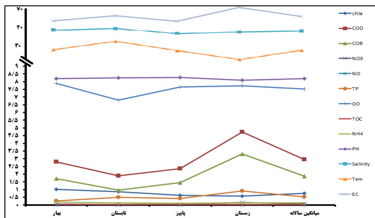
شکل ۲) مقایسه روند میانگین کلی غلظت فاکتورهای فیزیکی و شیمیایی آب در فصول مختلف، دما (درجه سانتی‌گراد)، pH (واحد استاندارد)، COD، BOD، نیترات، شوری، آمونیم، کل کربن آلی (برحسب میلی‌گرم بر لیتر)؛ DO (درصد اشباع)؛ EC (میکروزیمنیس بر سانتی‌متر)
