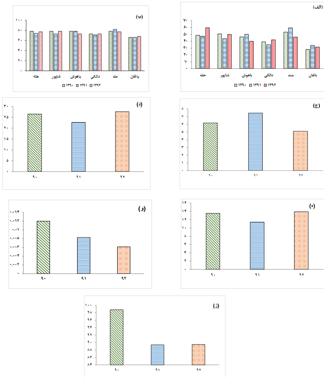
شکل ۲) مقایسه دو شاخص کیفیت آب و مقادیر پارامترهای کیفیت آب (الف) IRWQISC، (ب) NSFQI و (ج) NO 3 (mg/l) و (د) COD (mg/l)، (ه) BOD (mg/l) و (و) PO 4 (mg/l) و (ز) DO (%) در رودخانه‌های استان بوشهر در سال‌های ۹۰ تا ۹۲
