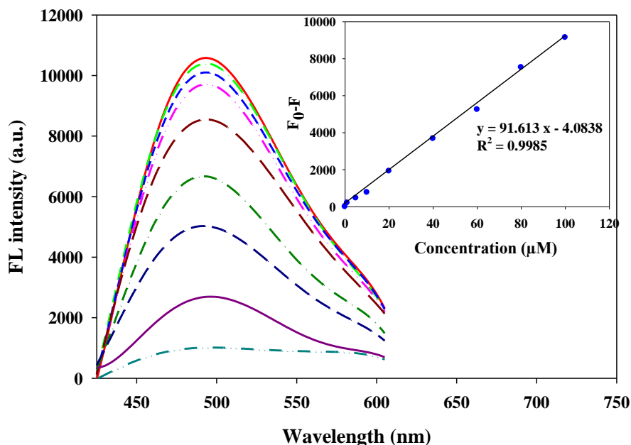
شکل ۷ طیف‌های نشر فلورسانس نانوذرات پلی دوپامین در حضور غلظت‌های مختلف گالیک اسید در محدوده ۰ تا ۱۰۰ میکرومولار. قسمت داخل: رابطه بین مقادیر کاهش شدت سیگنال فلورسانس ( F_0-F ) در برابر غلظت گالیک اسید (منحنی کالیبراسیون)
