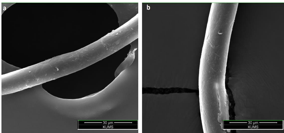
شکل ۵) تصویر میکروسکپ الکترونی از میکروپلاستیک‌های موجود در نمونه‌های تنه‌نشتی هوا
