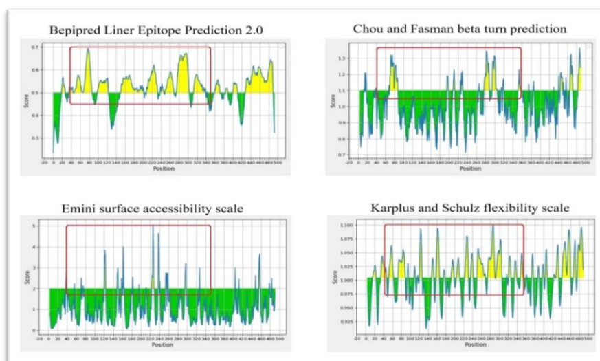
شکل ۱. نتایج آنالیز اپیتوپ‌های خطی B-Cell، با استفاده از الگوریتم‌های مختلف پروفایل اپیتوپی توالی آمینواسیدی TolC به دست آمد که ناحیه بین آمینواسیدهای ۴۰ تا ۳۳۵ (در نمودارها داخل کادر قرمز) بیشترین میزان اپی توپ را شامل می‌شد.
