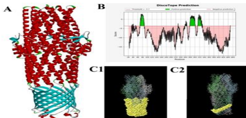
شکل ۲. بررسی اپی توپ‌های فضایی در پروتئین TolC، (A) ساختار سوم پیش‌بینی شده از پروتئین TolC از باکتری شینگلا فلکسنری، (B) اپیتوپ‌های فضایی با سرور DiscoTope فقط در سه ناحیه ۷۶-۹۰، ۲۸۰-۳۳۰ و ۳۱۰-۳۳۰ قرار داشت، (C) اپیتوپ‌های فضای پیش بینی شده با سرور ElliPro، C1 ۱۰۱ ناحیه با قدرت بالای اپیتوپی به رنگ زرد مشخص شده است، C2 قویترین اپیتوپ فضایی در ناحیه ۶۴-۹۳ به رنگ زرد مشخص شده است.
