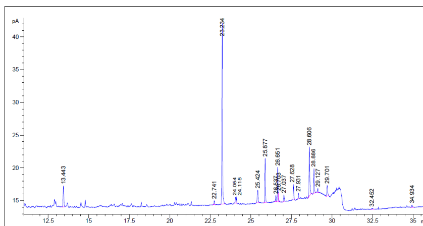
شکل ۲) یک کروماتوگرام مربوط به پروفایل اسیدهای چرب موجود در کاهوی دریایی ( Ulva lactuca ) سواحل پوشهر به روش GC-FID Fig. 2) A chromatogram associated with the fatty acid profile of the Ulva lactuca from the Busher coast by GC-FID method.
