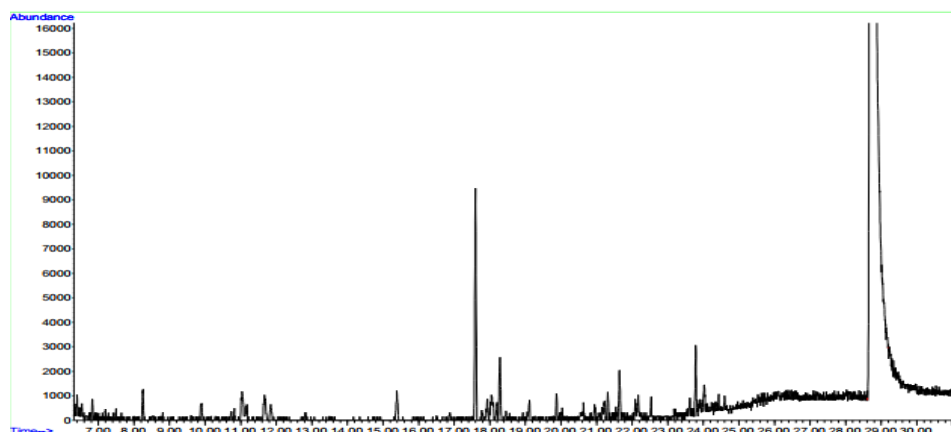
شکل (۵) کروماتوگرام مربوط به آنالیز ترکیبات شیمیایی کاهوی دریایی ( Ulva lactuca ) به دست آمده از سواحل بوشهر به روش GC-MS Fig. 5) chromatogram related to the chemical composition of the alga Ulva lactuca from the Bushehr coast by GC-MS method.
