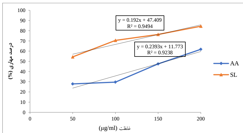
شکل (۶) فعالیت آنتی‌اکسیدانی کاهوی دریایی ( Ulva lactuca ) در مقایسه با استاندارد آسکوربیک اسید توسط روش DPPH Fig. 6) Antioxidant activity of Sea Lettuce (SL), compared to the ascorbic acid (AA) by DPPH method.
