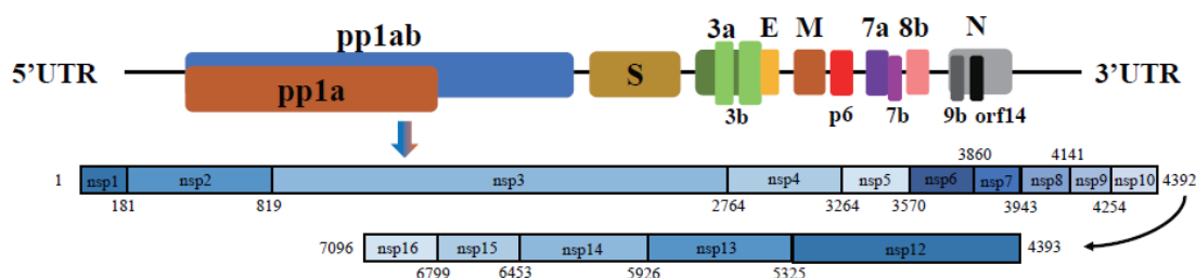
شکل (۱) سازمان بندی ژنوم کروناویروس جدید SARS-CoV-2
