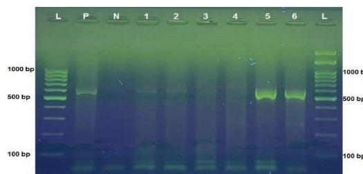
شکل ۲) الکتروفورز محصول PCR دور دوم کریپتوسپوریديوم 18S rRNA. L: نشانگر اندازه DNA 100b، P: کنترل مثبت؛ N: کنترل منفی؛ ۱-۶: نمونه‌ها
