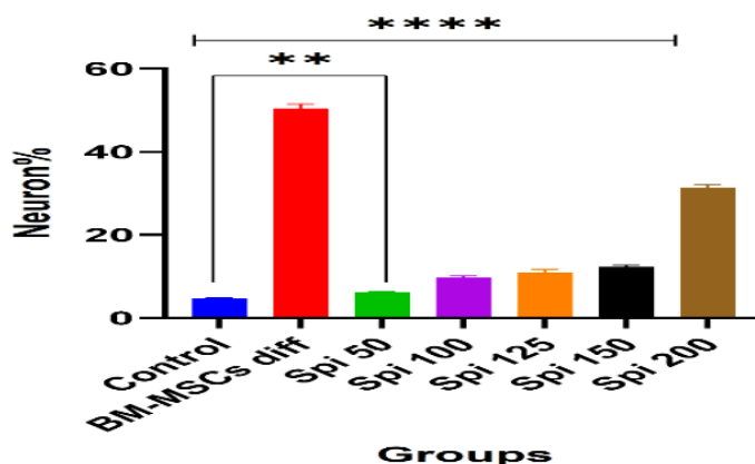
شکل ۴. میزان تمایز نورونی در گروه‌های دریافت‌کننده اسپیرولینا و مقایسه آن با گروه کنترل. داده‌ها بصورت میانگین \pm ارائه شده است. علامت ستاره نشان‌دهنده تفاوت معنی‌دار است. ****P < ۰/۰۰۰۰۱ , **P < ۰/۰۱
