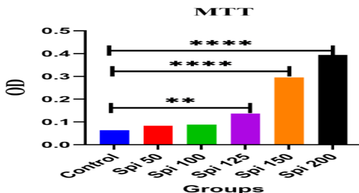
شکل ۲. بقای سلولی بین گروه‌های دریافت‌کننده عصاره اسپیرولینا و گروه کنترل، داده‌ها بصورت میانگین \pm ارائه شده است. علامت ستاره نشان‌دهنده تفاوت معنی‌دار است. **** P < 0.0001 ، ** P < 0.01
