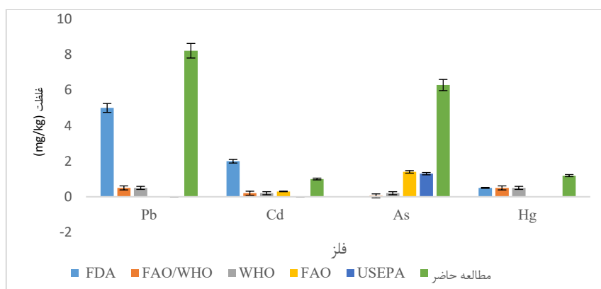
شکل ۴. مقایسه غلظت‌های فلزات سنگین در بافت عضله ماهیان مرکب با استانداردهای بین‌المللی (میلی‌گرم بر کیلوگرم) Fig 4. Comparison of Heavy Metal Concentrations in Squid Muscle Tissue with International Permissible Limits (mg/kg)
