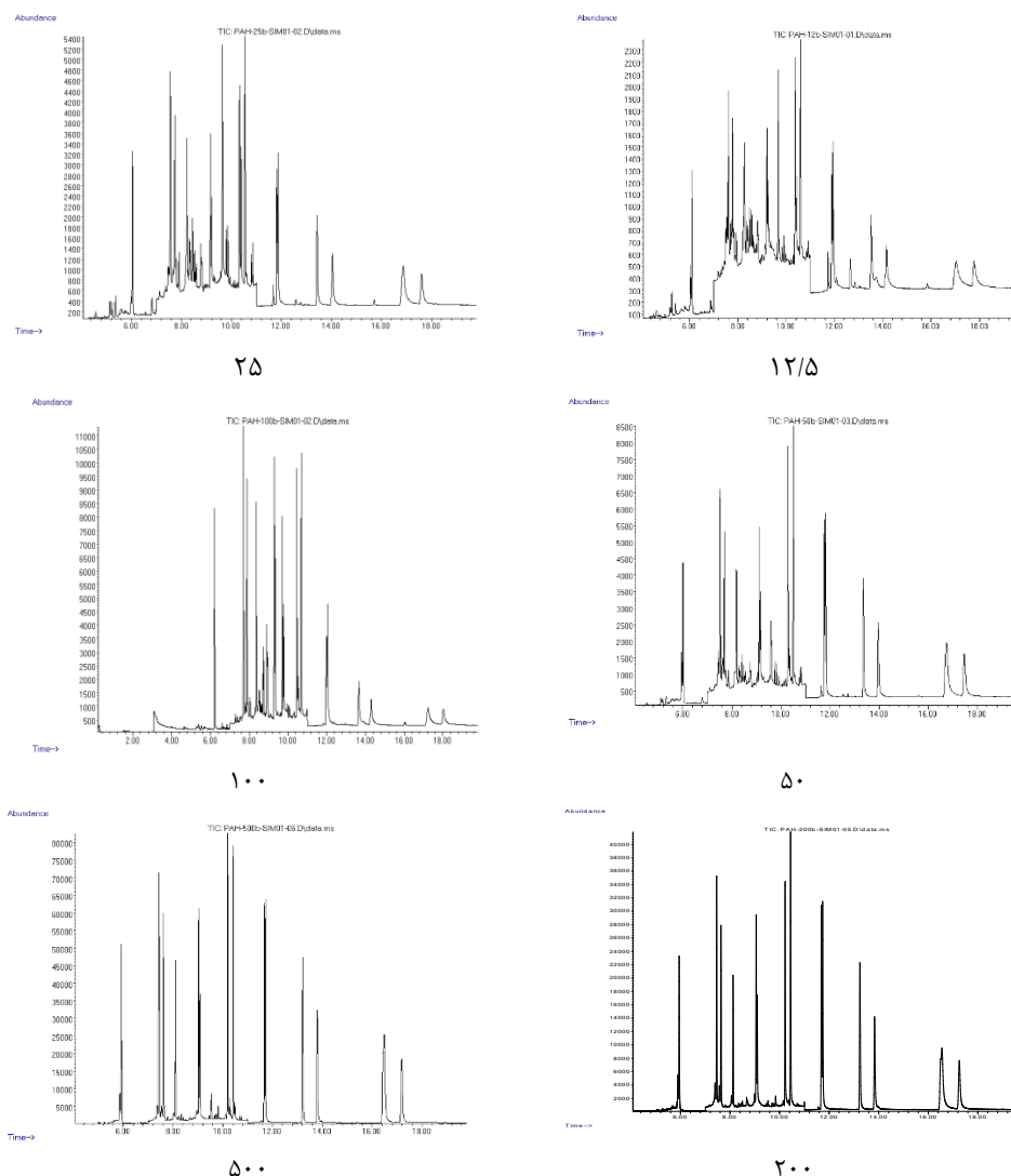
شکل ۱. کروماتوگرام‌های استاندارد حاصل از GC-MS، در محدوده غلظتی بین ۱۲/۵ تا ۵۰۰ میکروگرم بر کیلوگرم PAH Fig 1. GC-MS chromatograms of PAH standards at concentrations ranging from 12.5 to 500 µg/kg
