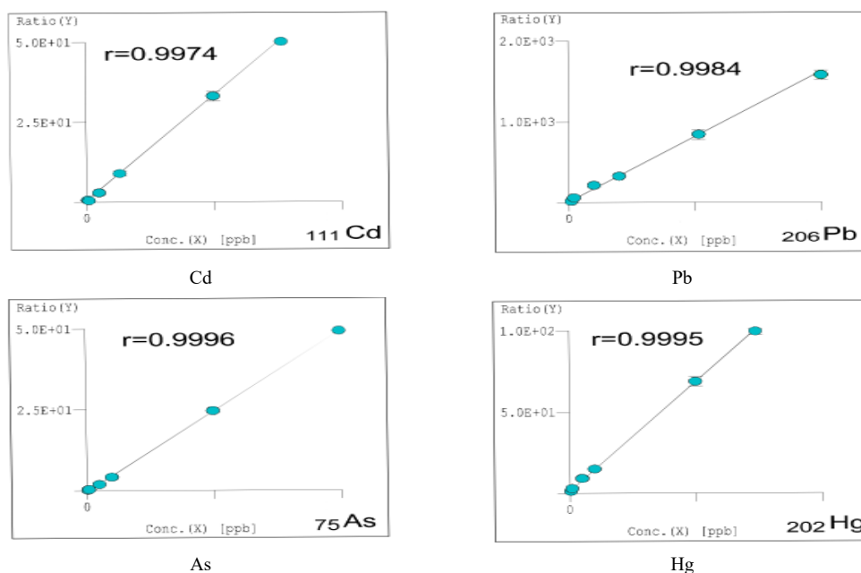
شکل ۳. منحنی‌های کالیبراسیون مربوط به فلزات سرب، آرسنیک، کادمیوم و جیوه در غلظت‌های ۰/۵، ۱، ۲، ۵ و ۱۰ میکروگرم بر کیلوگرم Fig 3. Calibration curves for lead, arsenic, cadmium, and mercury at concentrations of 0.5, 1, 2, 5, and 10 \mu\text{g/kg} .
