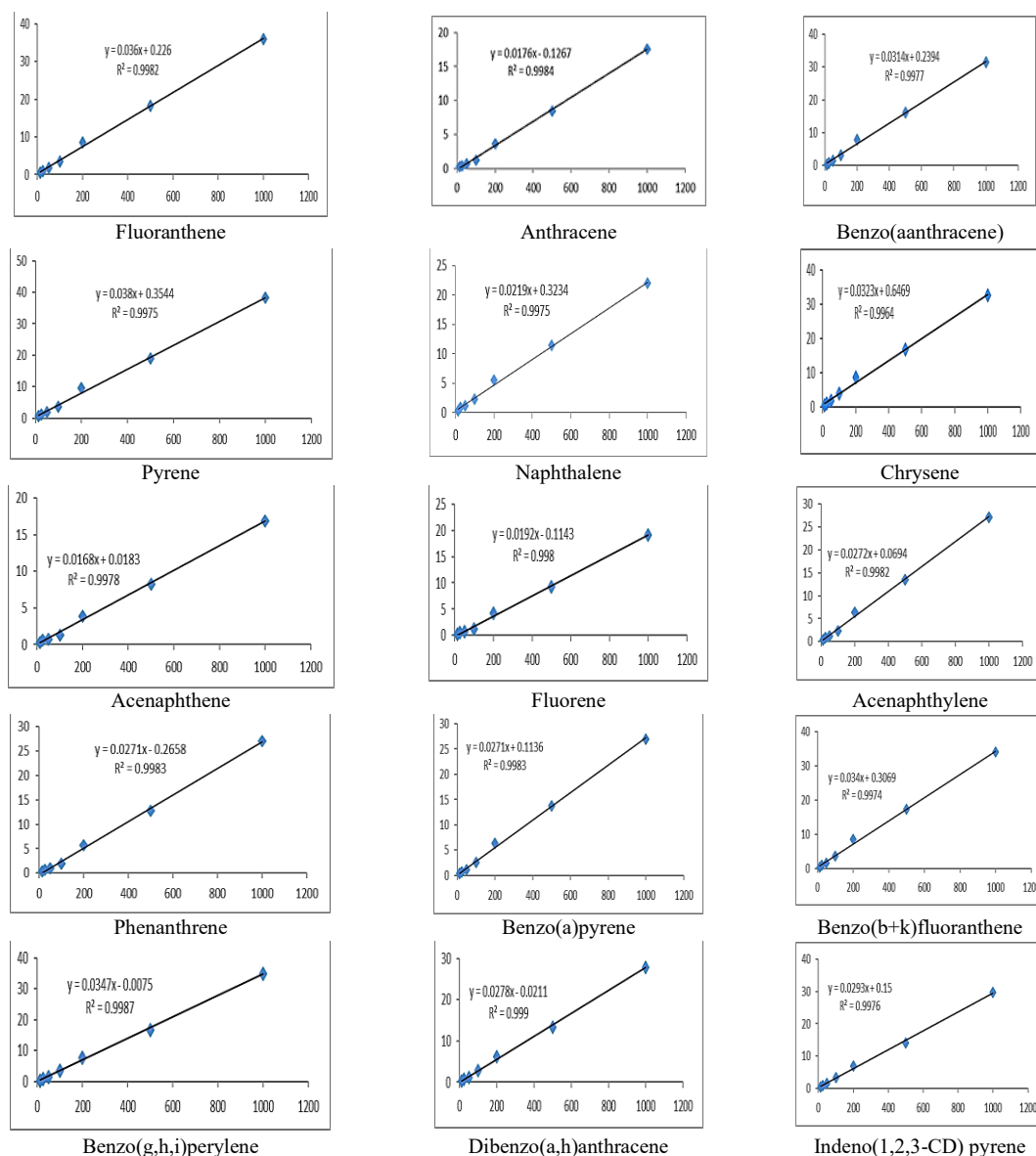
شکل ۲. منحنی‌های کالیبراسیون مربوط به هر هیدروکربن آروماتیک چندحلقه‌ای در غلظت‌های مختلف Fig 2. Calibration curves for each polycyclic aromatic hydrocarbon (PAH) at different concentrations
