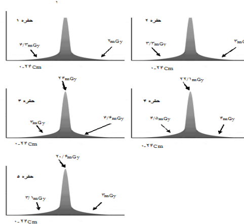
شکل ۲ الف) نمودارهای توزیع دُز بر حسب میلی گری در راستای محور Z برای نواحی سر
