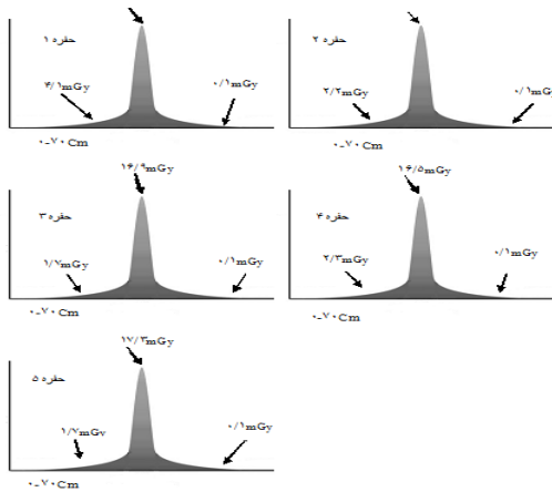
شکل ۲ ب) نمودارهای توزیع دُز بر حسب میلی گری در راستای محور Z برای نواحی تنه
