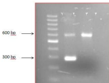
شکل ۳ ژل الکتروفورز حاصل از واکنش AS-PCR کدون KatG ۳۱۵ . از سمت چپ ستون (۱): مارکر (۱۰۰ bp)، ستون (۲): شامل باند مادر ۶۲۰ bp و باند ۲۹۰ bp مربوط به یک نمونه حساس به ایزونیاژید، ستون (۳): فقط شامل باند مادر ۶۲۰ bp مربوط به نمونه مقاوم به ایزونیاژید، ستون (۴): کنترل منفی (فاقد DNA)
