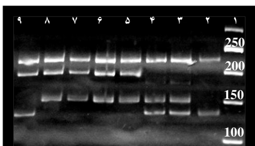
شکل ۲ (A, B, C, D) الگوهای PCR-RFLP در نمونه‌های حساس و مقاوم به ایزونیاژید. از سمت راست ستون (۱): مارکر (۵۰ bp)، ستون (۲): نمونه مقاوم به ایزونیاژید با الگوی C، ستون (۳ و ۴): نمونه‌های حساس به ایزونیاژید با الگوی A، ستون (۵ تا ۸): نمونه‌های حساس به ایزونیاژید با الگوی B، ستون (۹): نمونه مقاوم به ایزونیاژید با الگوی D
