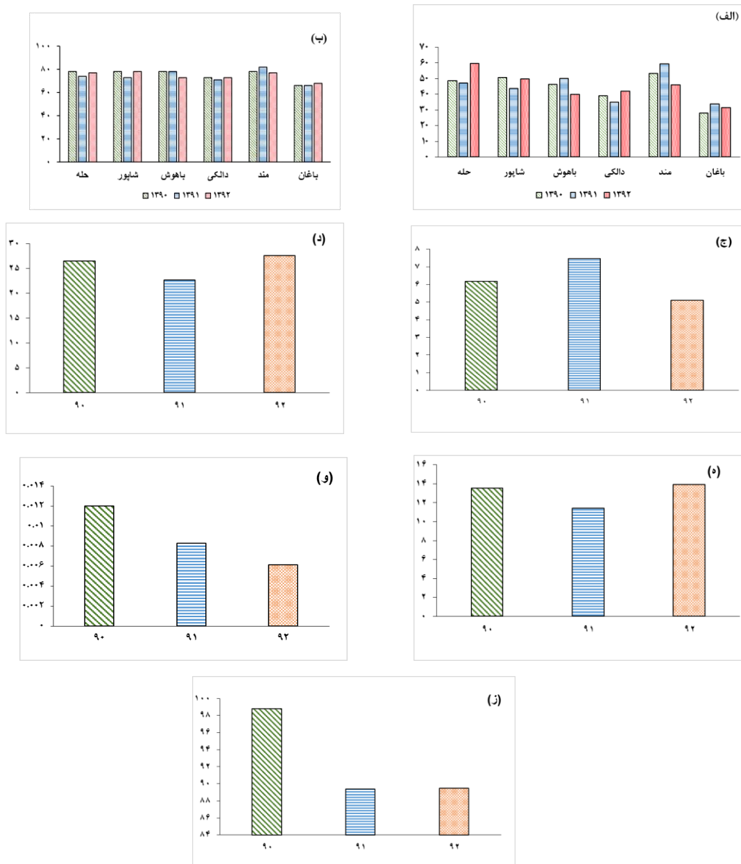
شکل ۲) مقایسه دو شاخص کیفیت آب و مقادیر پارامترهای کیفیت آب (الف) IRWQISC, (ب) NSFQI, (ج) NO 3 (mg/l) و (د) COD (mg/l), (ه) BOD (mg/l), (و) PO 4 (mg/l) و (ز) DO (%) در رودخانه‌های استان بوشهر در سال‌های ۹۰ تا ۹۲
