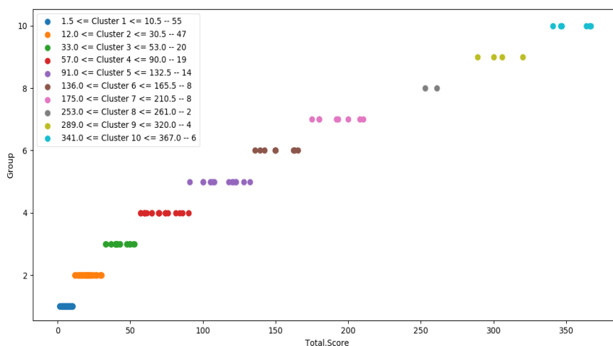
شکل ۳) خوشه بندی دهگانه داده ها با حذف صفر و بزرگتر از ۳۶۷ Fig 3) Decuple clustering of data by removing 0 and a score greater than 367
