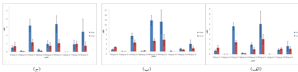
شکل ۱) مقایسه‌ی میانگین غلظت عناصر در عضله و پوست میگوهای صید شده از بندرگاه
