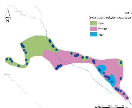
شکل ۲) توزیع مکانی غلظت نیترات برحسب میلی‌گرم بر لیتر چاه‌های مورد مطالعه
