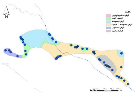
شکل ۵) نقشه نهایی توزیع مکانی کیفیت شیمیایی آب‌های زیرزمینی منطقه مورد مطالعه
