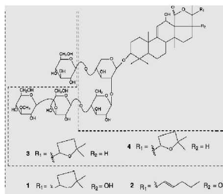
شکل ۵ ساختارهای مولکولی هولتورین های A, B, C و D از خيار دریایی Holothuria forskali
