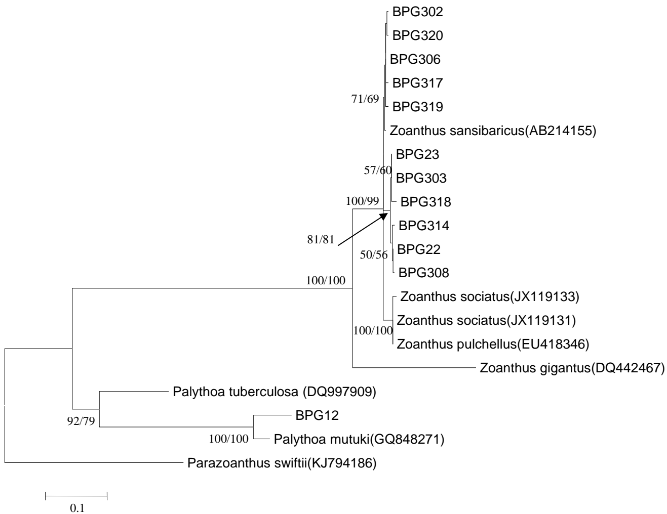
شکل 5: درخت Maximum likelihood بر اساس قطعه ژنی ITS rDNA شامل توالی‌های جدید حاصل از مطالعه حاضر و توالی‌های پیشین ثبت شده در بانک ژن. ارزش‌های بوت استرپ به ترتیب برای ML و NJ روی گره‌ها نشان داده شده‌است.
